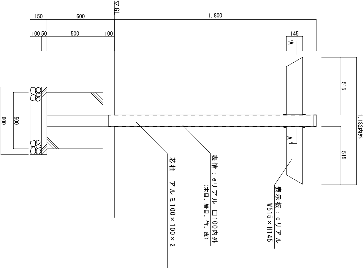
正面図 S=1:20
